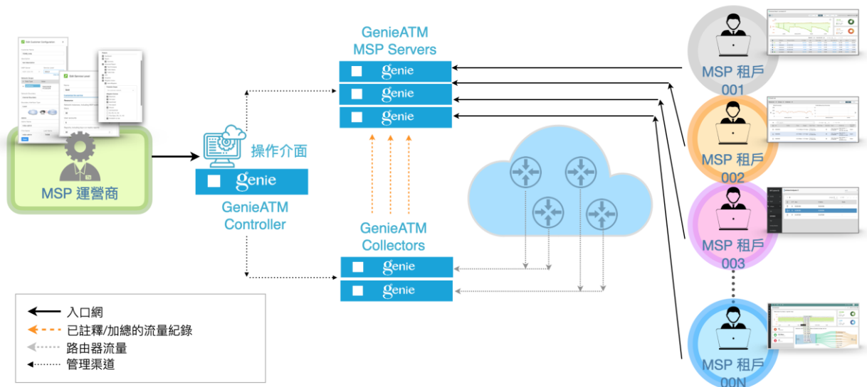
GenieATM MSP Server產品流程圖
